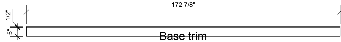
1 front Scale: 3/8" = 1'-0"
